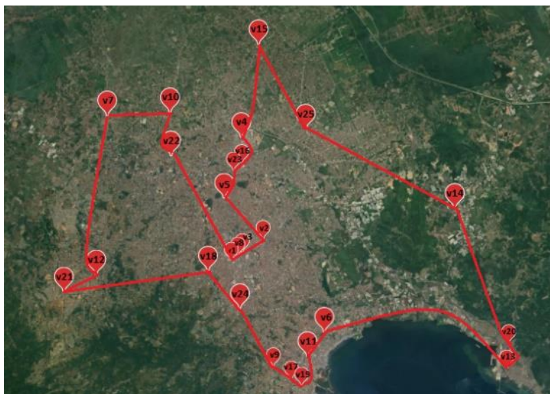
Gambar 13. Tour yang didapat dari opsi kedua setelah dilakukan revisi tour .
