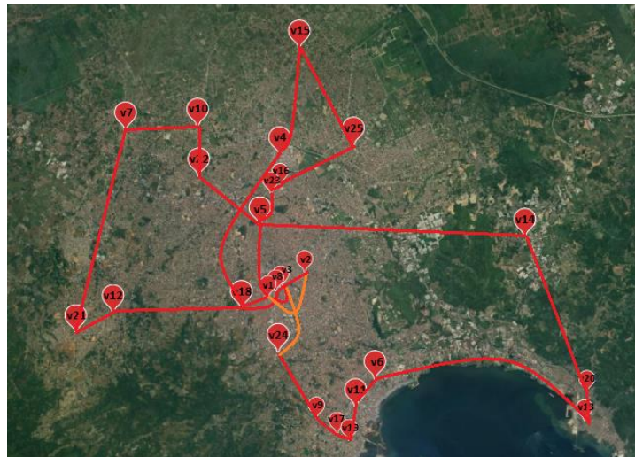
Gambar 8. Hasil yang didapat pada opsi pertama setelah titik v_9 berderajat 2.
